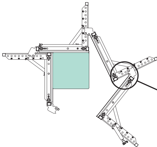
2. Ecarter également du béton le deuxième élément. Bloquer les deux éléments en « position d'ouverture bloquée » à l'aide de deux broches supplémentaires (voir détail).
