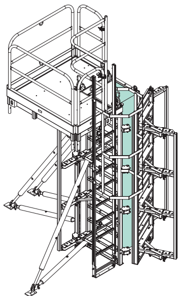
1. Dévisser les pièces de fermeture et déplier le premier élément poteau.
