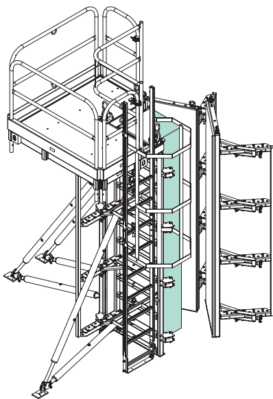
2. Ecarter également du béton le deuxième élément. Bloquer les deux éléments en « position d'ouverture bloquée » à l'aide de deux broches supplémentaires (voir détail).
